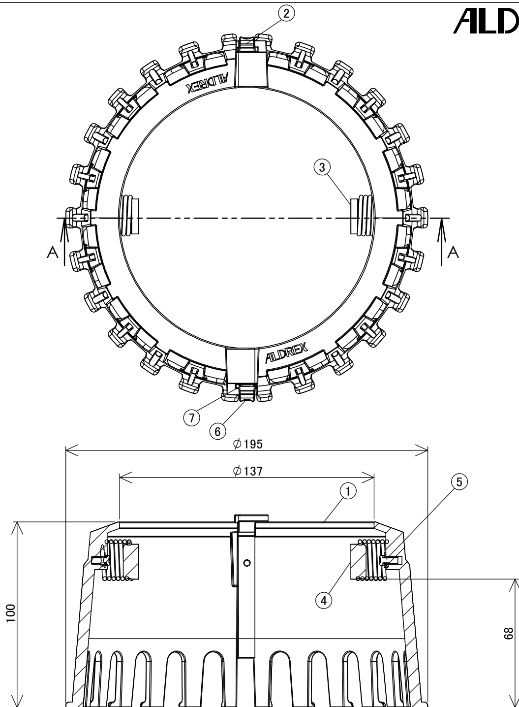
断面図 A-A
