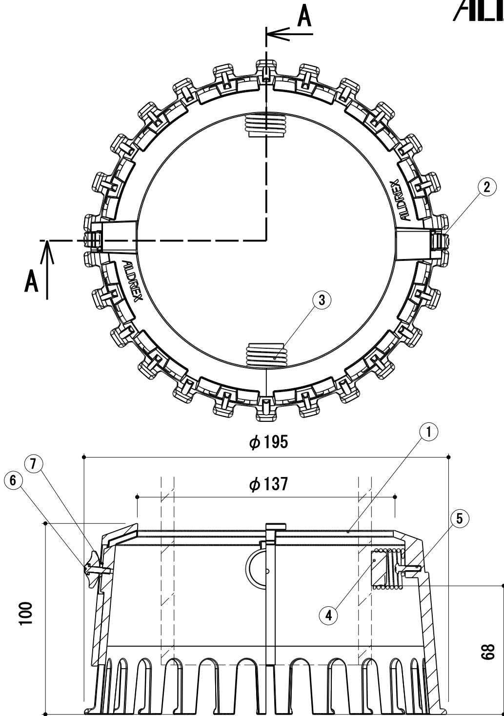
断面図A-A
