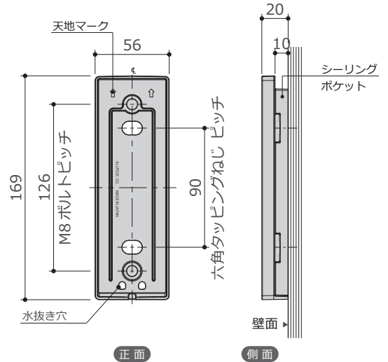
《シーリングポケット用固定プレート》 取付穴寸法
