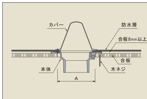
取付開口寸法
