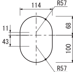
DY15型 防水シートカット寸法図
