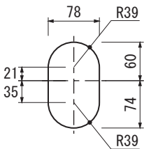
DY11型 防水シートカット寸法図
