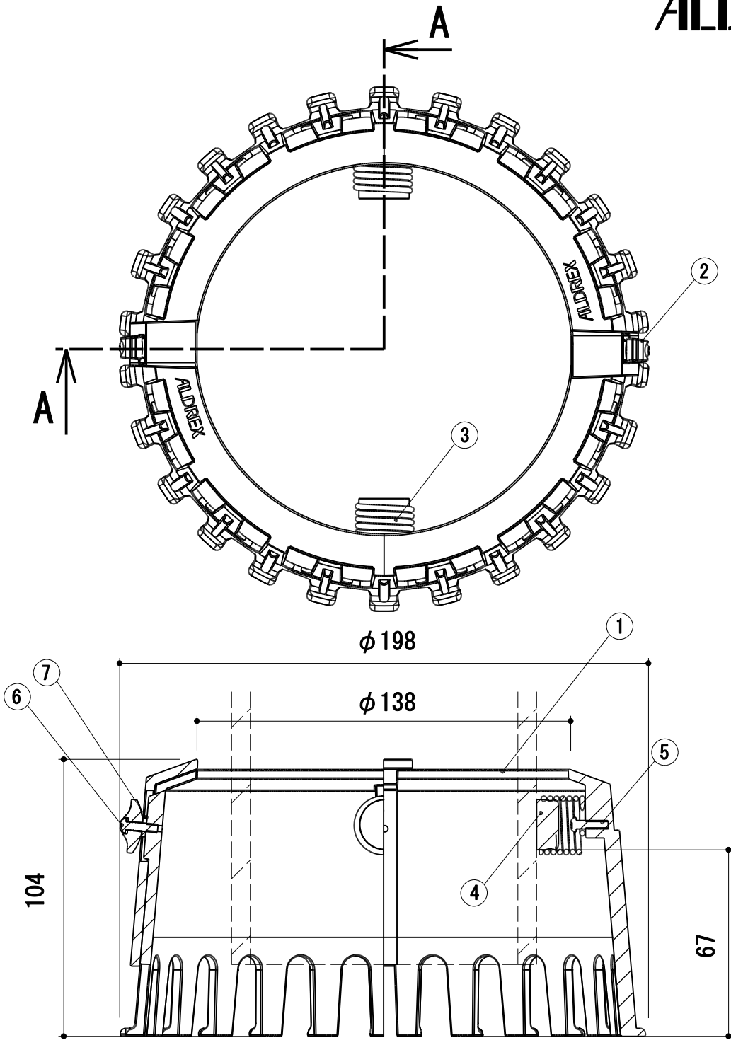
断面図A-A
